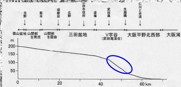
図6 武庫川の河川縦断面図。 横軸は篠山盆地南部における礫山川との谷中分水界からの水平距離を、縦軸は河床高度を示す。
