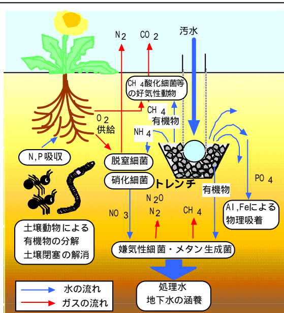
土壌トレンチ内における汚水の浄化機構
